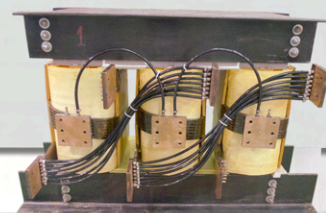
水冷式變壓器
